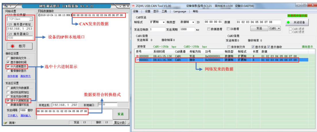
图 1.2.2 CAN 与网络数据透传
